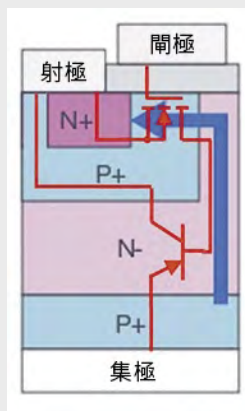
IGBT 切面圖
