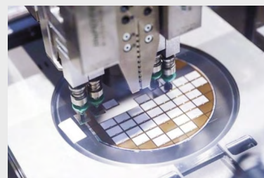
IGBT 芯片
